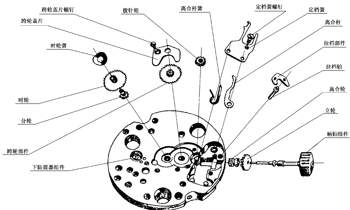
图 B.3 基础机心 表盘面 1
