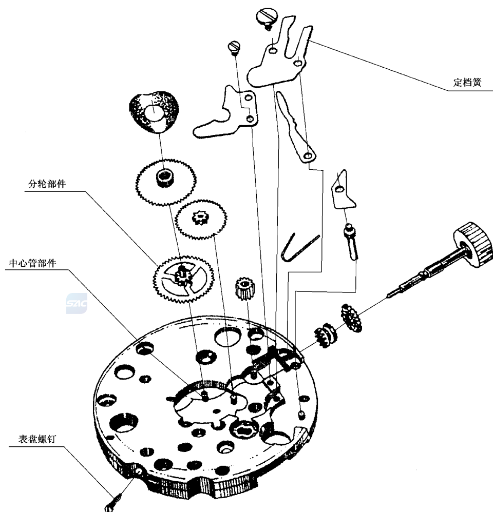
图 B.4 基础机心 表盘面 2
