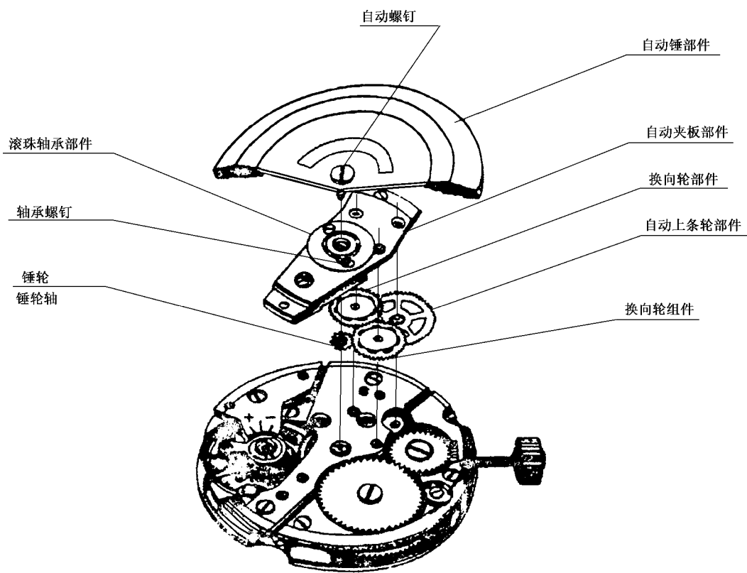
图 B.6 自动机构
