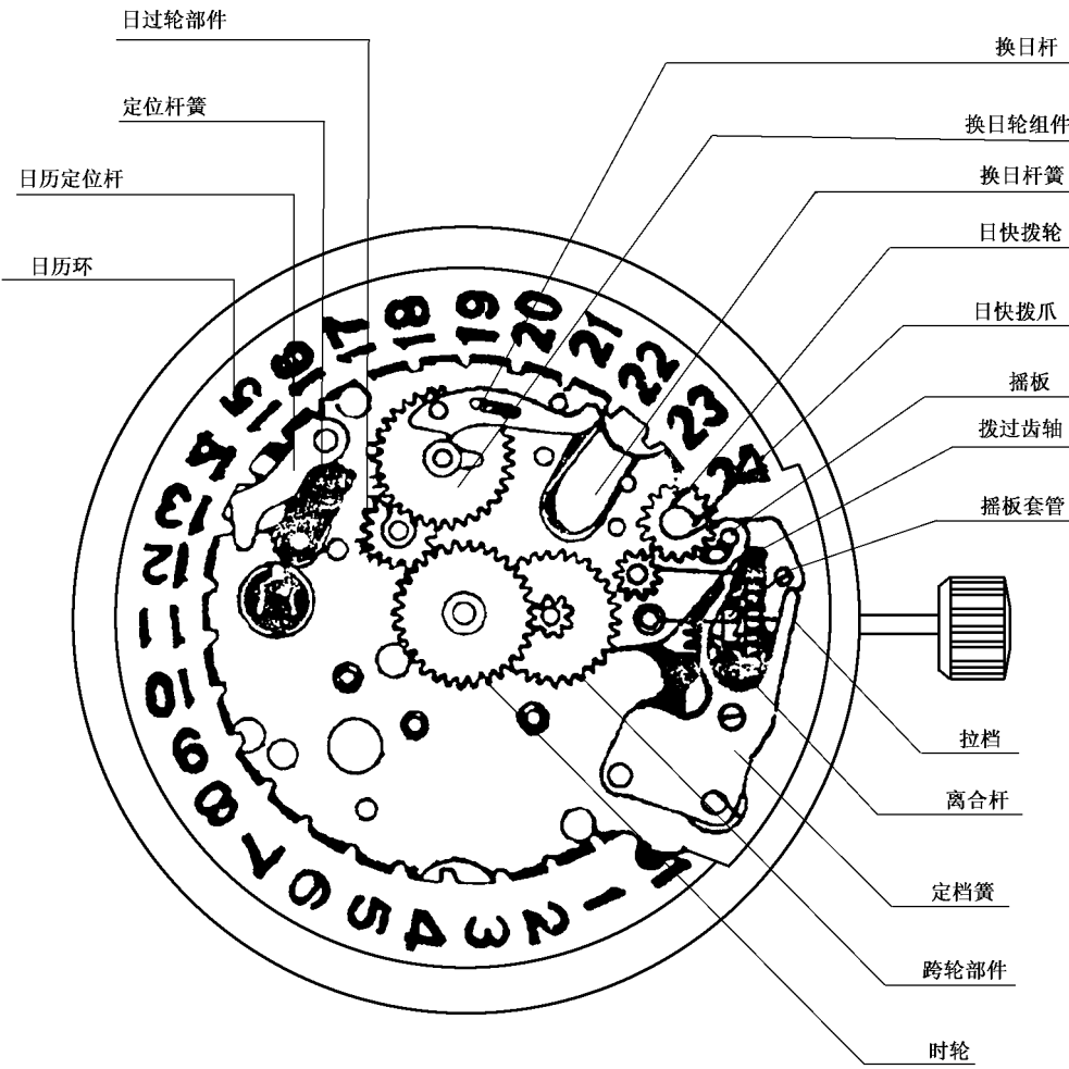
图 B.5 日历机构
