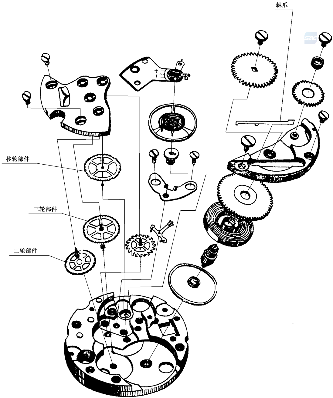
图 B.2 基础机心 偏二轮
