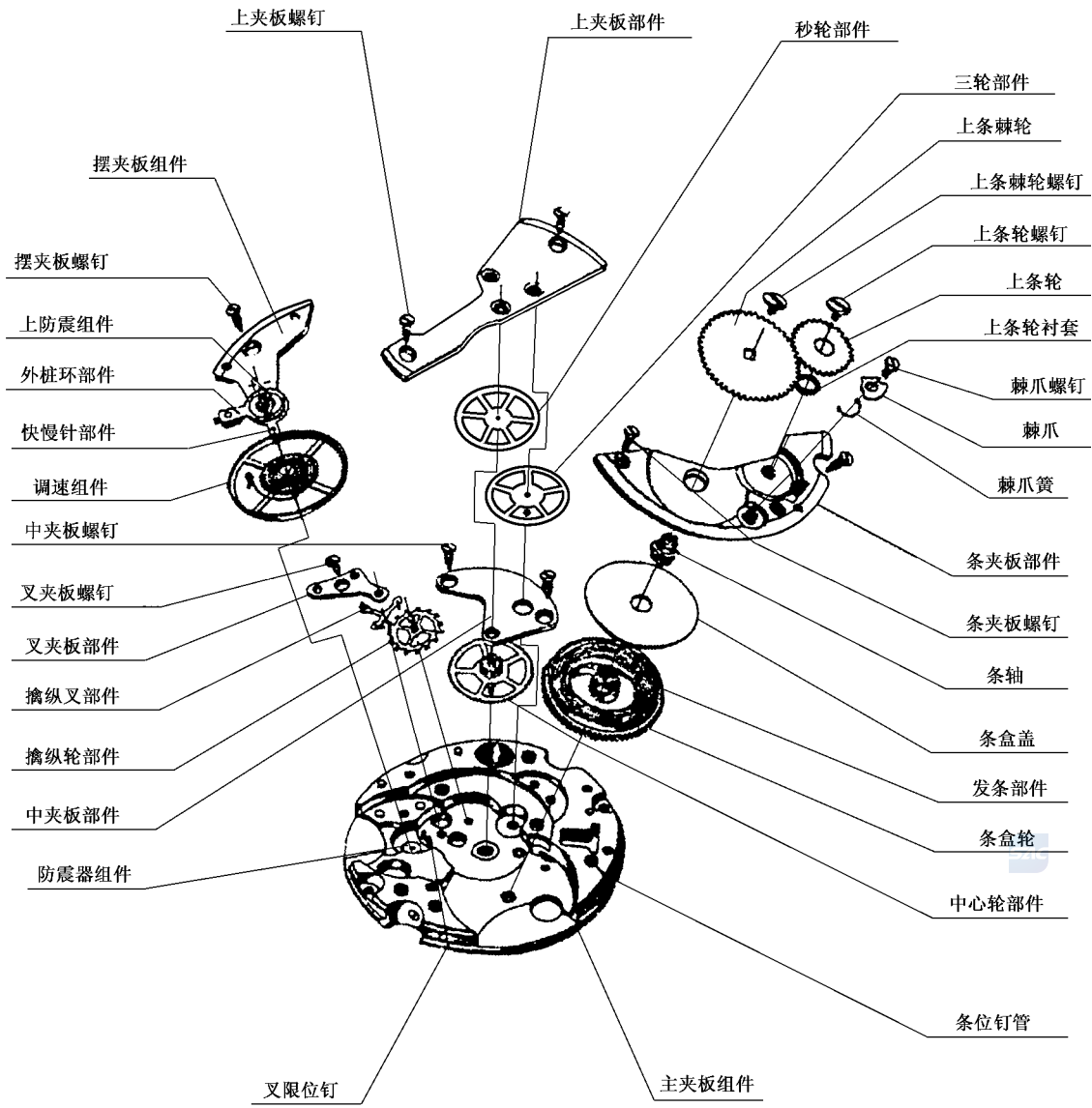
图 B.1 基础机心 直传式
